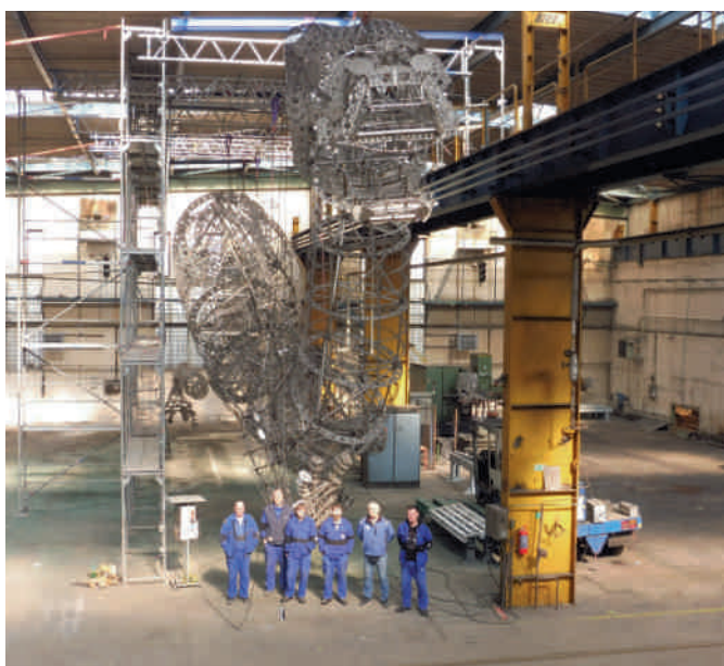
Cvičné sestavení konstrukce ještě na území ČR
